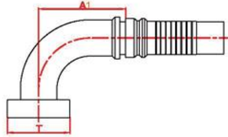
Kalın Flanşlı (SAE 6000) 45°- 90° Sıyrılmalı Hortum Rakorları
