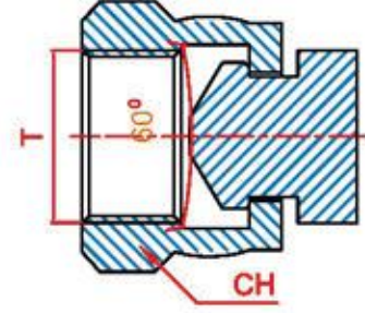
BSP Dişi Tapalar
